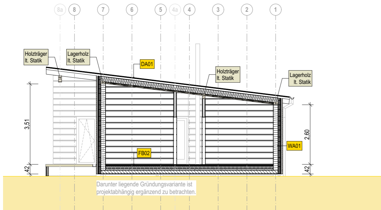
Schnitt 1
