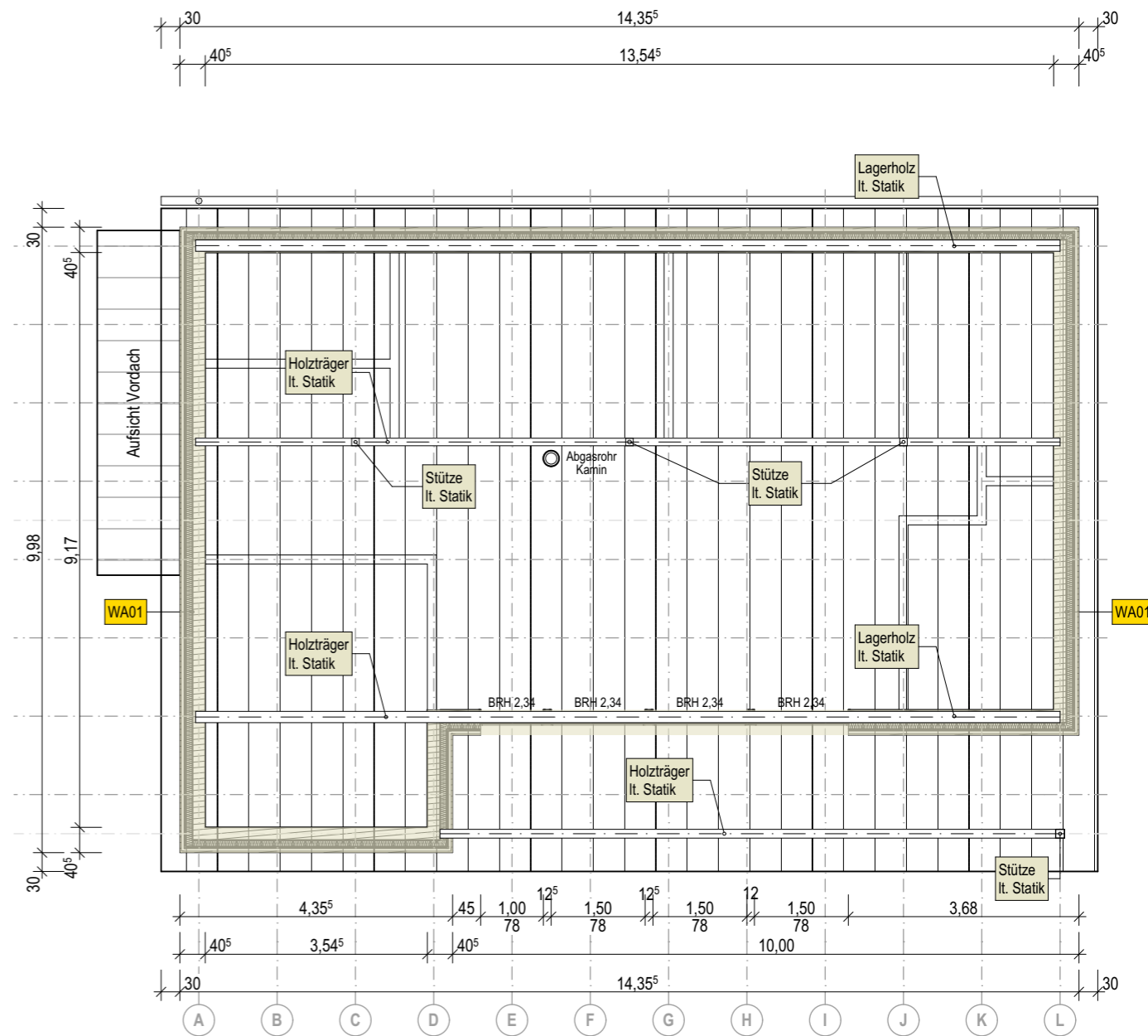
Grundriss Dach
