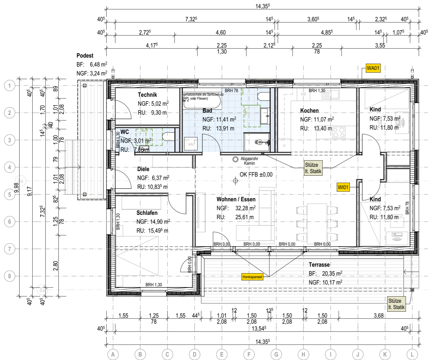
Grundriss EG
