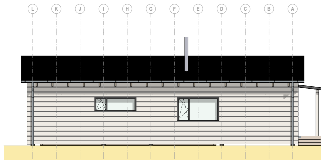
Ansicht 3
