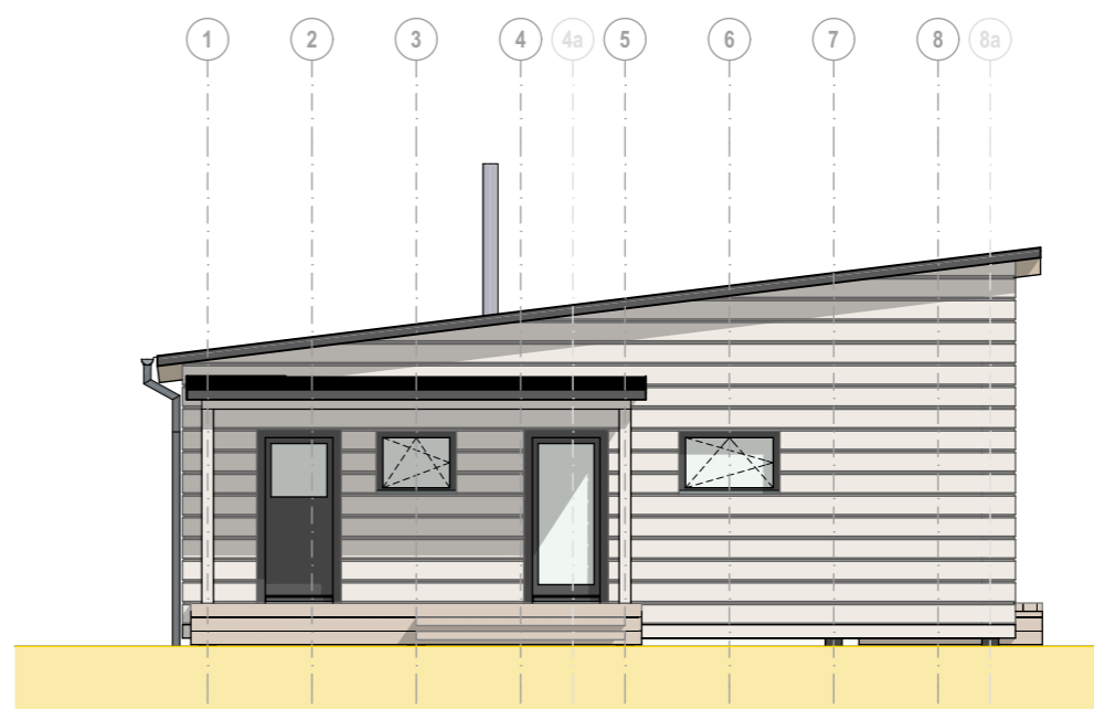
Ansicht 4
