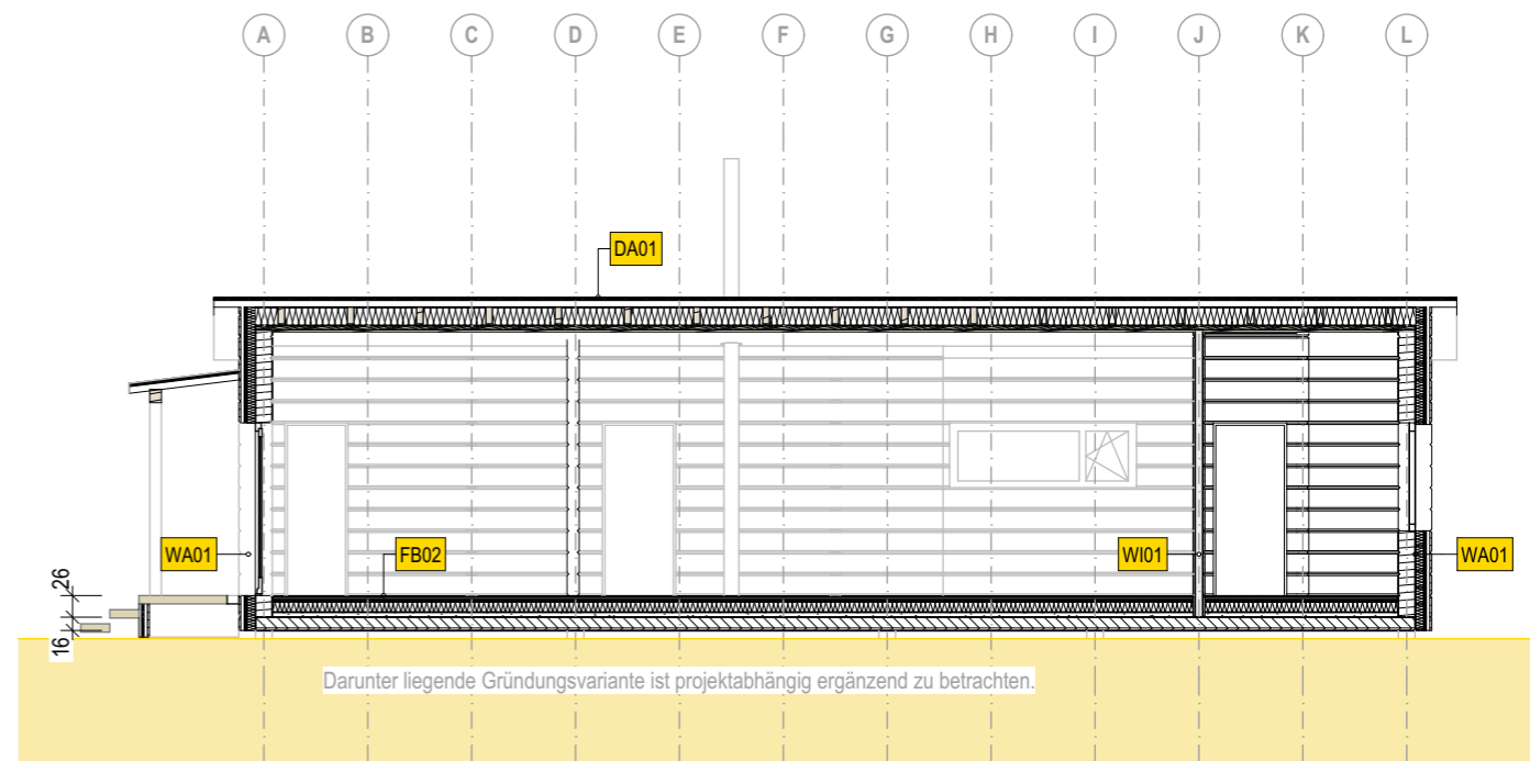
Schnitt 2
