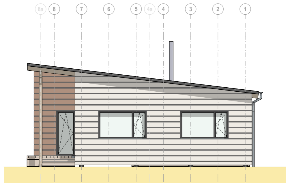
Ansicht 2
